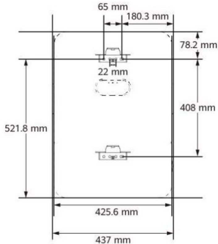
寸法(付属の背面取り付けブラケット)
