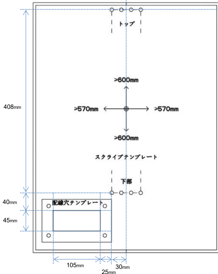
けがきテンプレート
