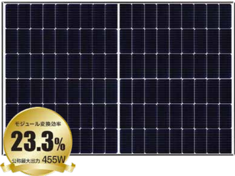
XLN108-455X 外形寸法:1722×1134×30mm
