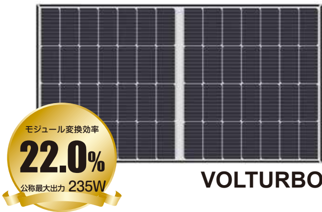
XLN56-235SC 外形寸法:1390×768×30mm
