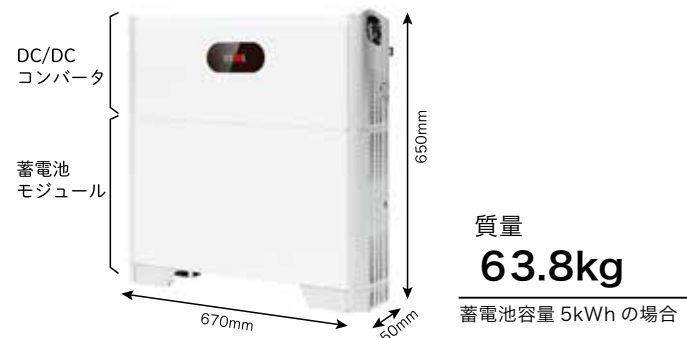
蓄電池システム (蓄電池モジュール、DC/DC コンバータ)
