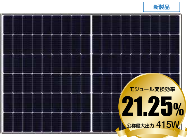
XLM108-415X 外形寸法:1722×1134×30mm
