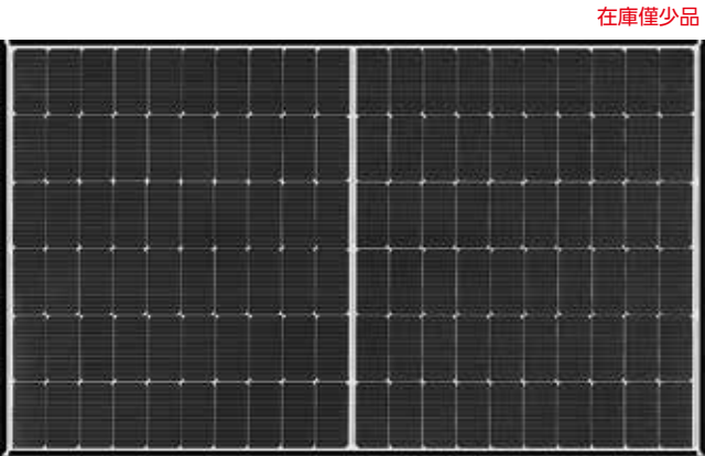
XLM120-380L <在庫については、お問い合わせください> 外形寸法:1755×1038×35mm
