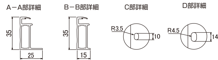
図 面 (単位:mm)
